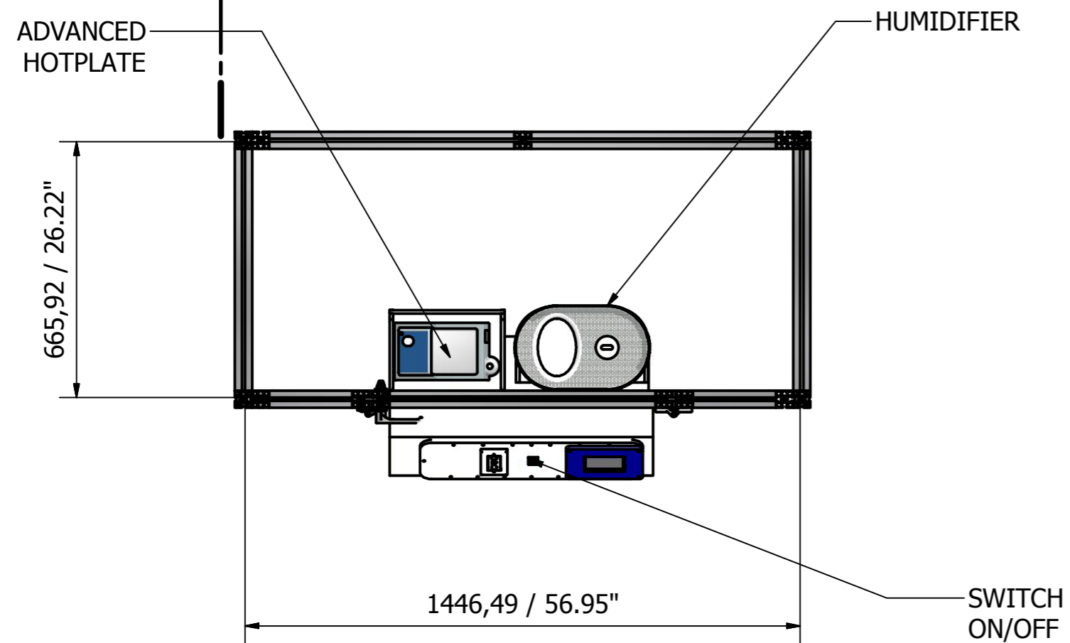
A-A ( 1 : 14 )
